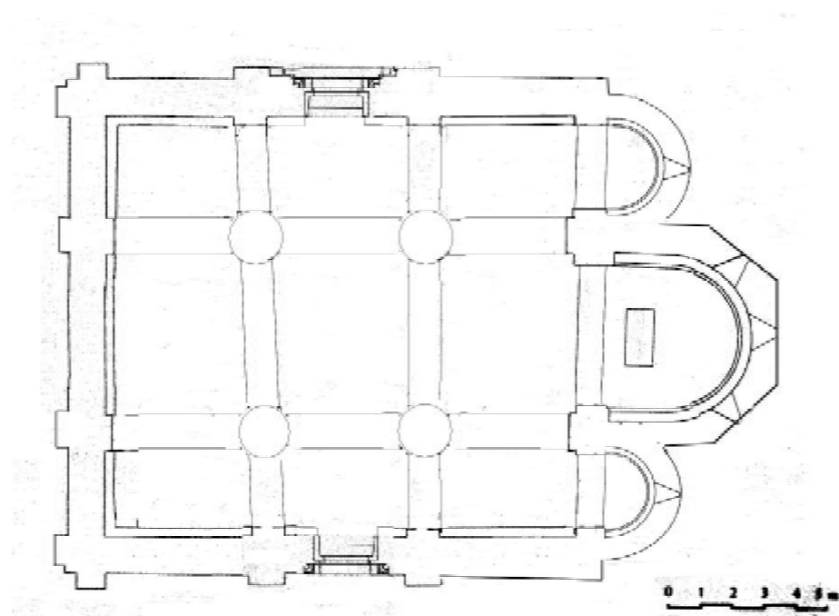
Fig.39 .- San Nicolás de Sangüesa. Croquis hipotético de su planta.
